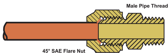
45° SAE Flare Nut
